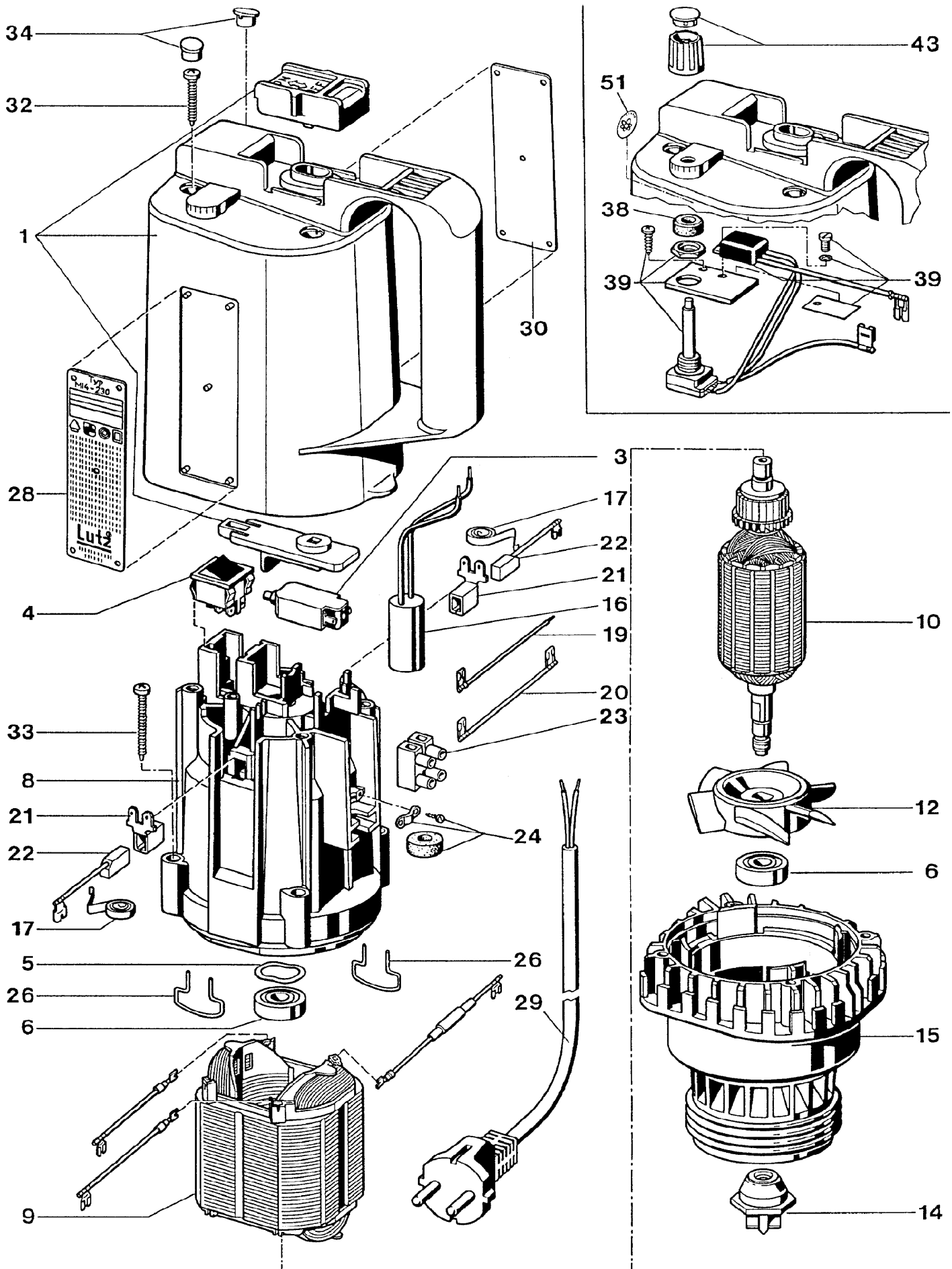
Motor MI 4-230 Motor MI 4-230 E Techn. Stand 01/03
